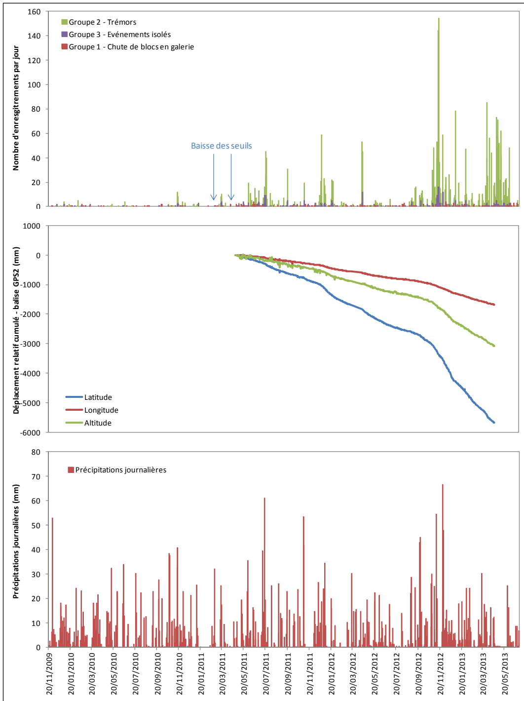
Figure 2. Activité microsismique journalière, déplacement cumulé à la balise GPS-RTK 2 et précipitations journalières du 20/11/2009 au 30/06/2013. La balise GPS-RTK 2 a été installée fin avril 2011 et déplacée fin avril 2013.
